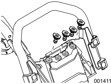
Figura 2-3. Inserción de las boquillas
