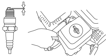
Figure 4-8. Bougie d'allumage
